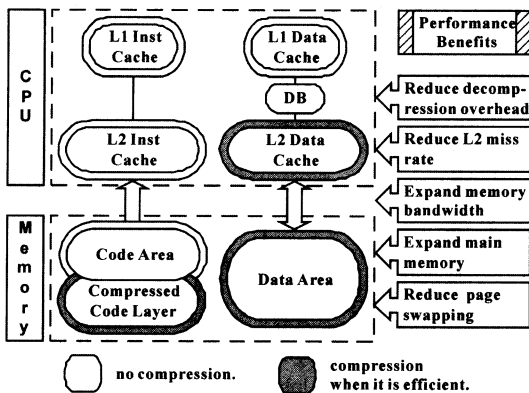
그림 3 HMCS의 전체구조와 성능상의 이득
