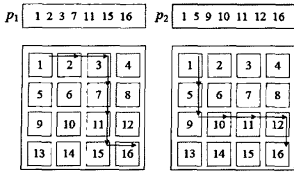
그림 6 라우팅 경로 인코딩
