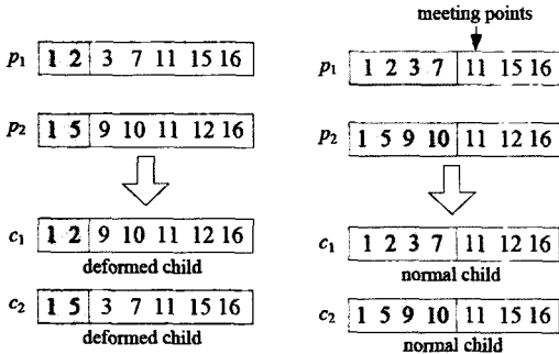
(a) one-point crossover (b) coordinate crossover 그림 7 라우팅을 위한 교차 연산
