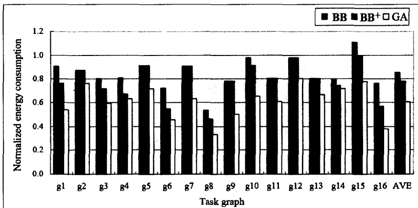
그림 13 B&B와 GA 기반 기법의 성능 비교
