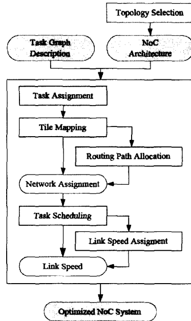
그림 3 저전력 NoC 시스템을 위한 설계 흐름
