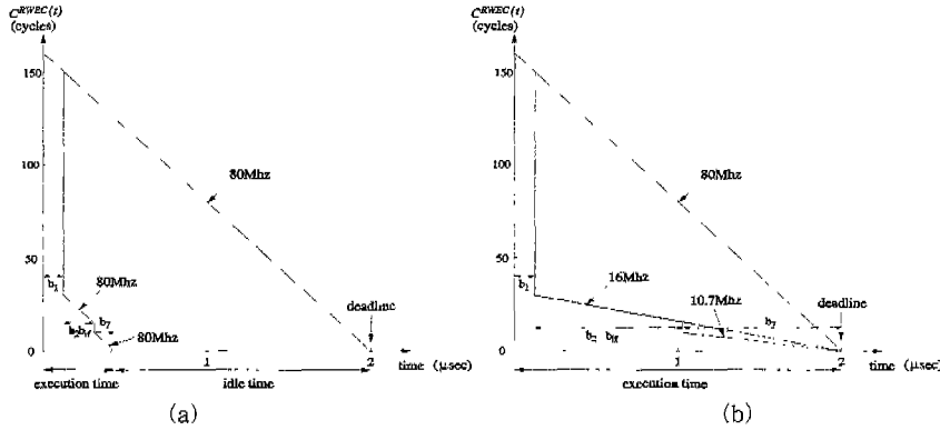
그림 4 속도 조정 알고리즘에 따른 C^{RWEC}(t) 의 변화: (a) 태스크내 스케줄링을 사용하지 않은 경우, (b) RWEC를 이용한 태스크내 스케줄링을 사용한 경우
