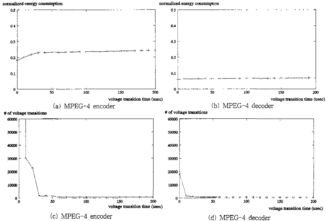
그림 8 AVS에 의해 변환된 MPEG-4 부호기와 복호기 프로그램의 정규화된 전력 소모값과 전압 조정 회수
